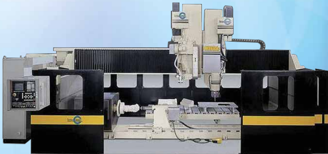
CNC Sústruh OMAG Lathe 94TE
