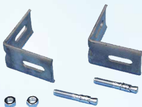
Montážny uholník Upínacia kotva M6 Upínacia kotva M8
