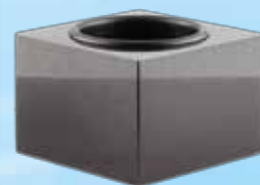
M33
